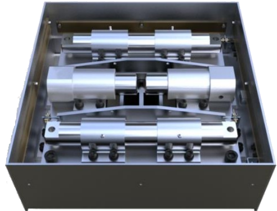
Robuster Aufbau
